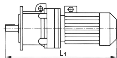
Исполнение на фланце
